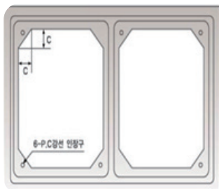
PC암거 2련 박스 예시
