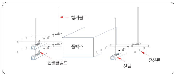
폴박스(노출 천장) 설치도
