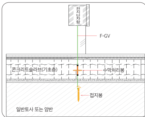
설치도면
