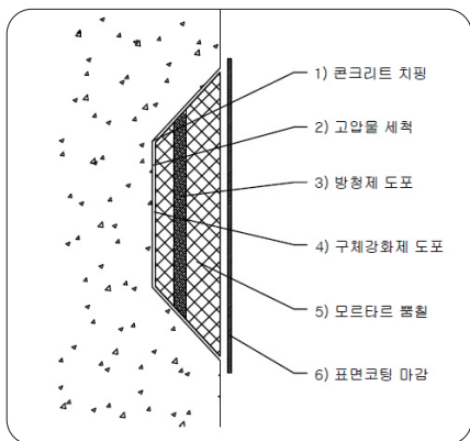
시공순서(철근노출 콘크리트)
