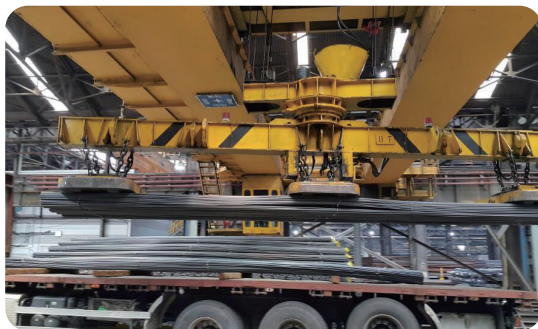
공장상차 작업(철근)
