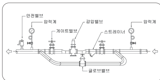
설치도
