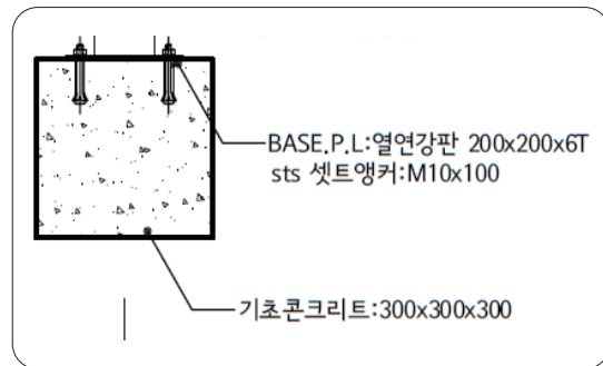
설치도면
