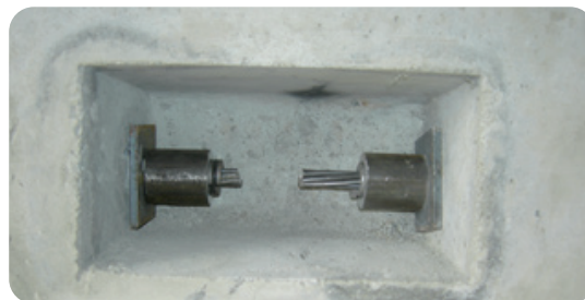
PC강선 조립완료(정착구)
