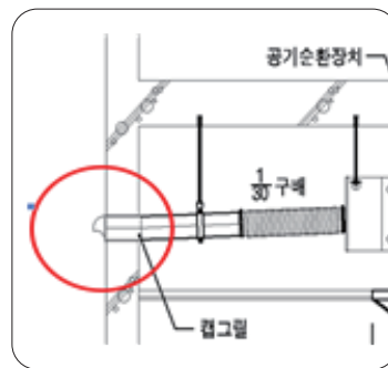
설치 형태
