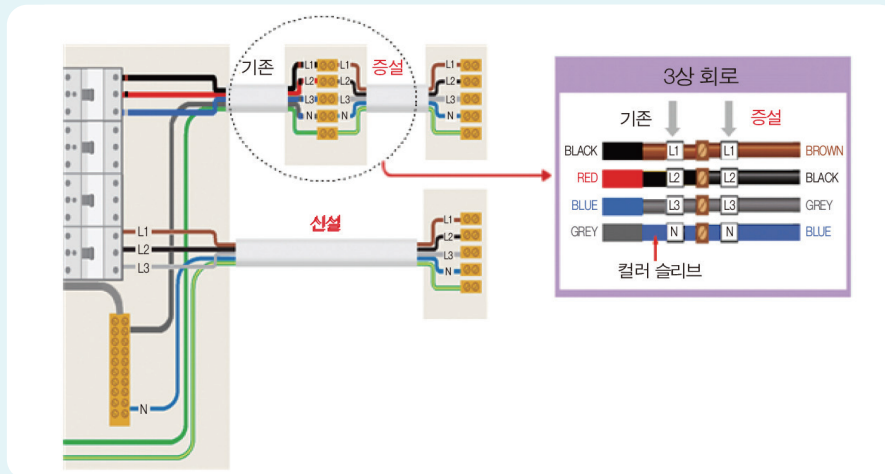
[그림] 전선 식별 변경 전후 - 증설 및 신설 적용 예시
