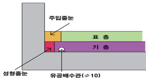
물빠기공 설치단면도
