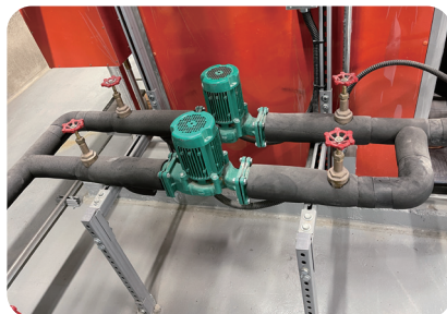
설치사진
